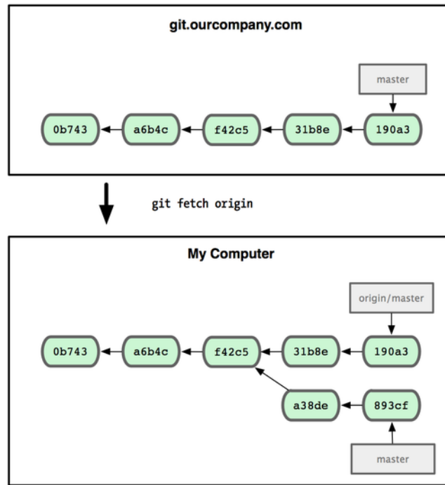
Figure 3.24: La commande git fetch met à jour vos références distantes.
