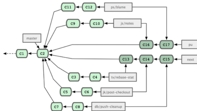
Figure 5.25: Fusion des branches thématiques dans les branches à long terme.
