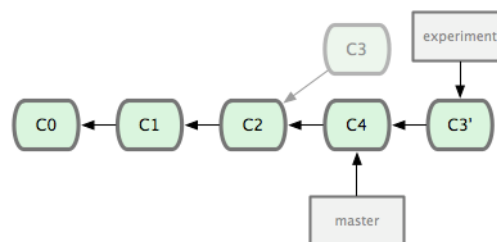
Figure 3.29: Rebaser les modifications introduites par C3 sur C4.
