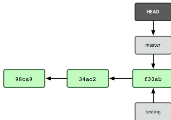
Figure 3.5: fichier HEAD pointant sur la branche active
