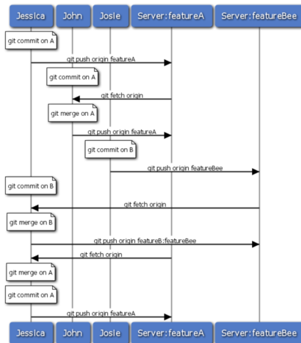
Figure 5.15: Une séquence simple de gestion orientée équipe.
