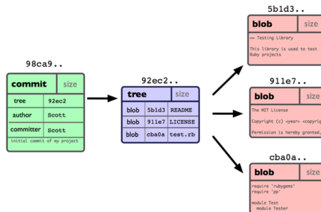
Figure 3.1: Données d'un unique commit.
