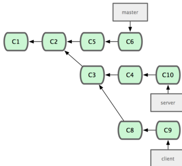
Figure 3.31: Un historique avec une branche qui sort d'une autre branche de sujet.
