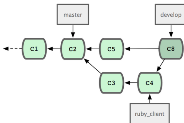
Figure 5.22: Après la fusion d'une branche thématique.
