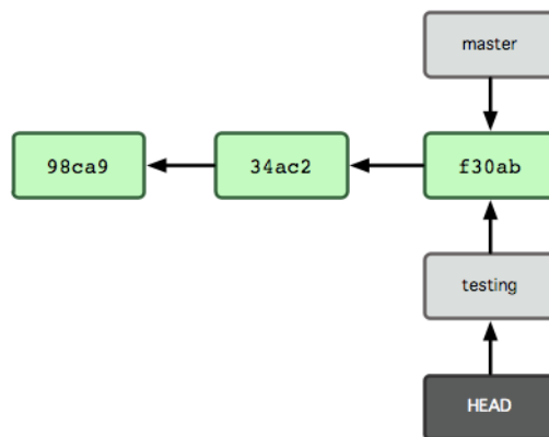
Figure 3.6: HEAD pointe vers une autre branche quand on bascule de branche
