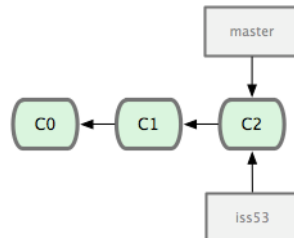
Figure 3.11: Création d'un nouveau pointeur de branche.
