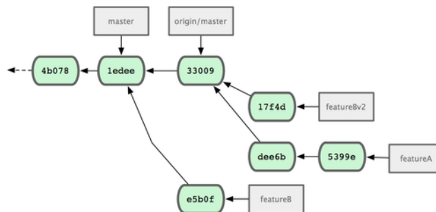
Figure 5.18: Historique des validations après le travail sur fonctionBv2 .
