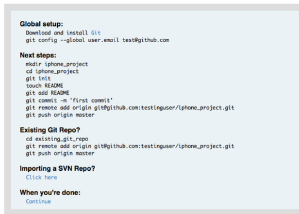
Figure 4.7: Instructions pour un nouveau dépôt
