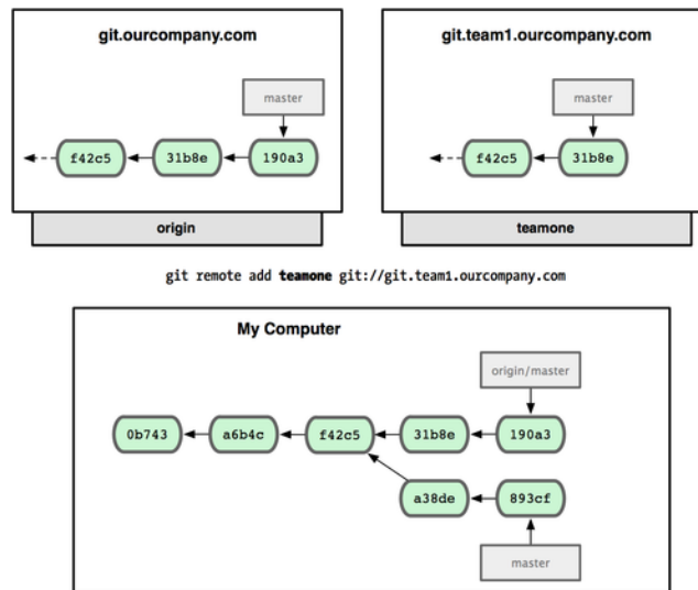
Figure 3.25: Ajouter un autre serveur comme accès distant.
