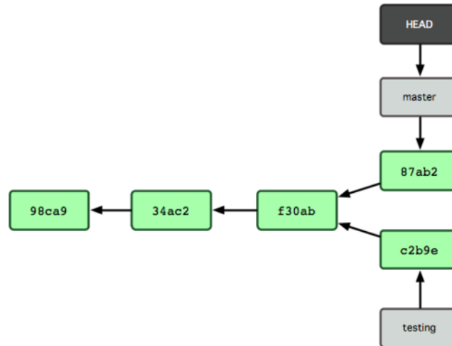
Figure 3.9: Les historiques de branche ont divergé.
