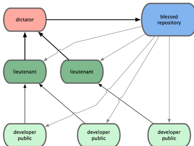
Figure 5.3: Le processus du dictateur bénévole.
