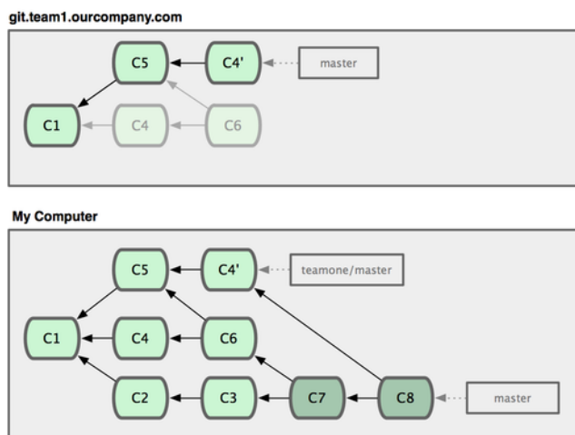
Figure 3.39: Vous fusionnez le même travail une nouvelle fois dans un nouveau commit de fusion.
