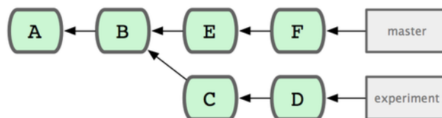
Figure 6.1: Exemple d'historique pour la sélection de plages de commits.
