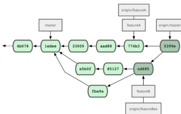
Figure 5.14: L'historique de Jessica après la fusion de ses deux branches thématiques.
