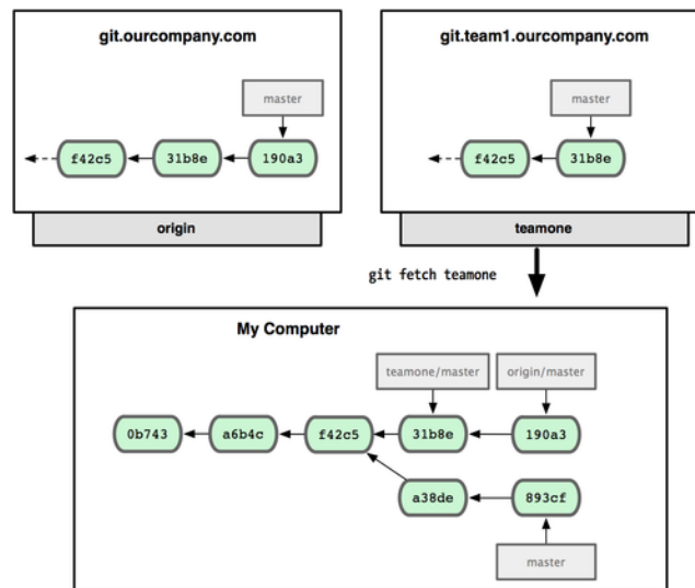
Figure 3.26: Vous récupérez une référence locale à la branch master de equipeun.
