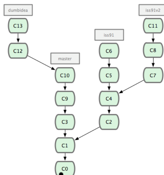
Figure 3.20: Votre historique de commit avec de multiples branches de sujet.
