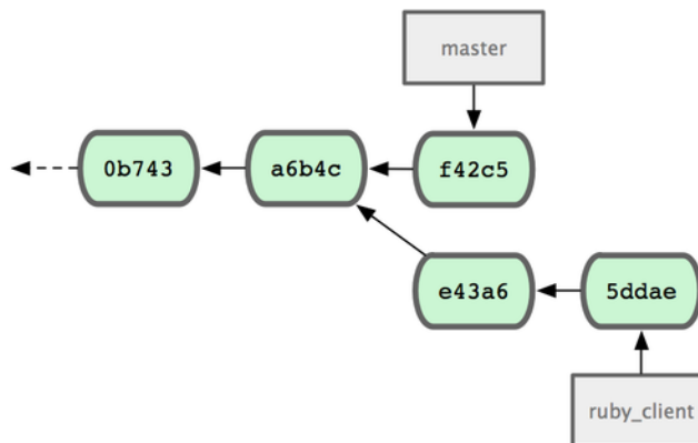
Figure 5.26: Historique d'exemple avant une sélection.
