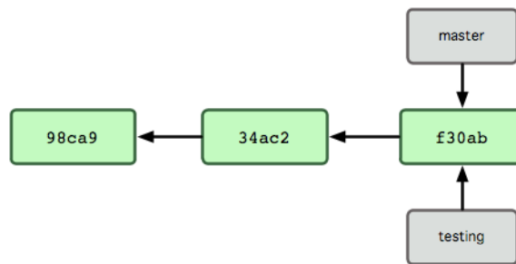
Figure 3.4: Branches multiples pointant dans l'historique des données de commit.
