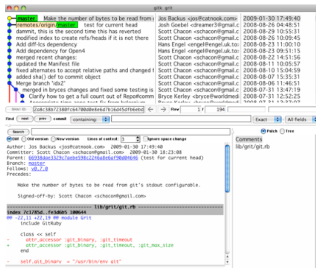
Figure 2.2: Le visualiseur d'historique gitk
