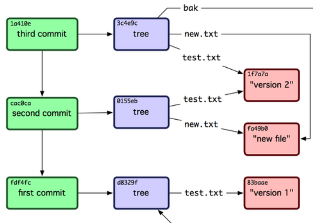
Figure 9.3: Tous les objets de votre répertoire Git.
