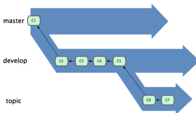
Figure 3.19: Représentation des branches comme des silos.
