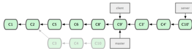
Figure 3.34: Rebase la branche server sur le sommet de la branche master .
