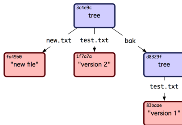
Figure 9.2: Structure des données actuelles de Git???
