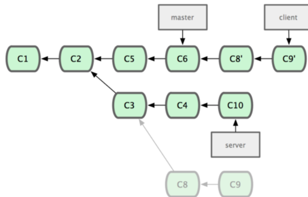
Figure 3.32: Rebaser une branche de sujet sur une autre branche.
