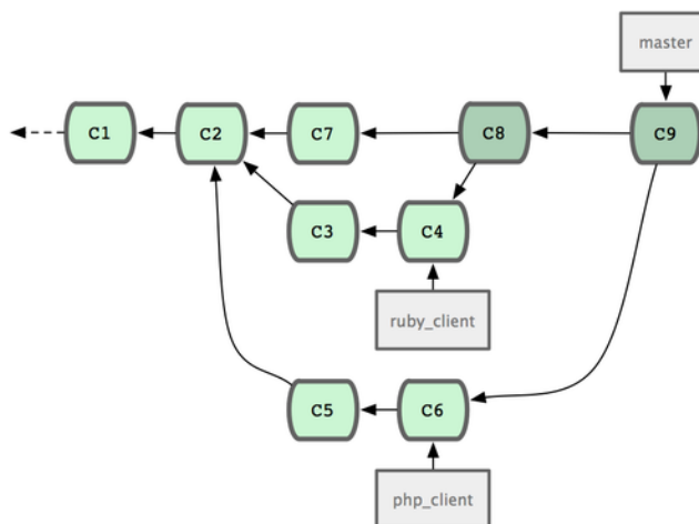
Figure 5.20: Après fusion d'une branche thématique.
