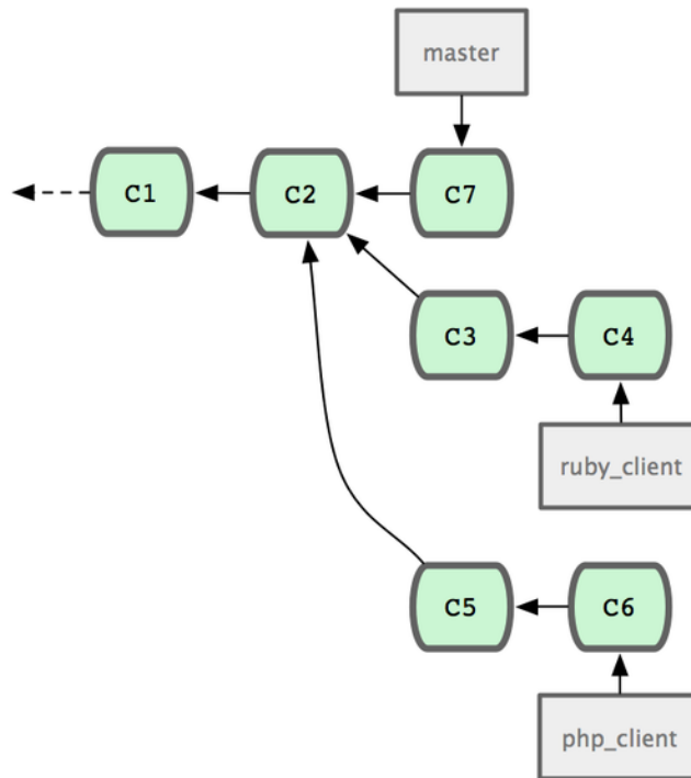
Figure 5.19: Historique avec quelques branches thématiques.
