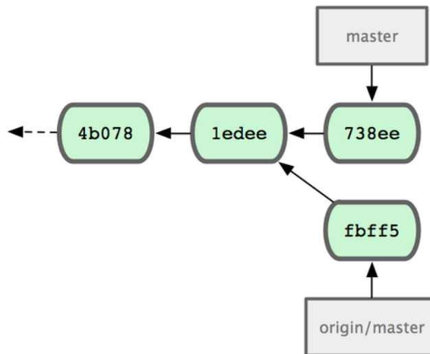
Figure 5.4: État initial du dépôt de John.
