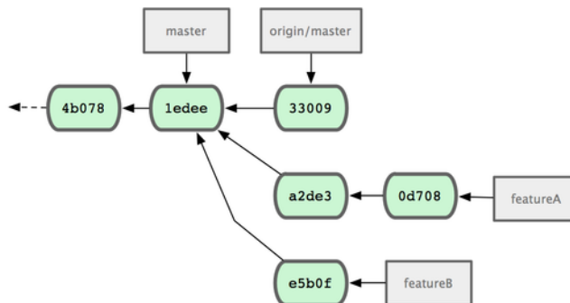
Figure 5.16: Historique initial des commits avec les modification de fonctionB.
