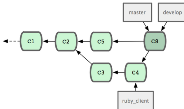
Figure 5.23: Après une publication d'une branche thématique.
