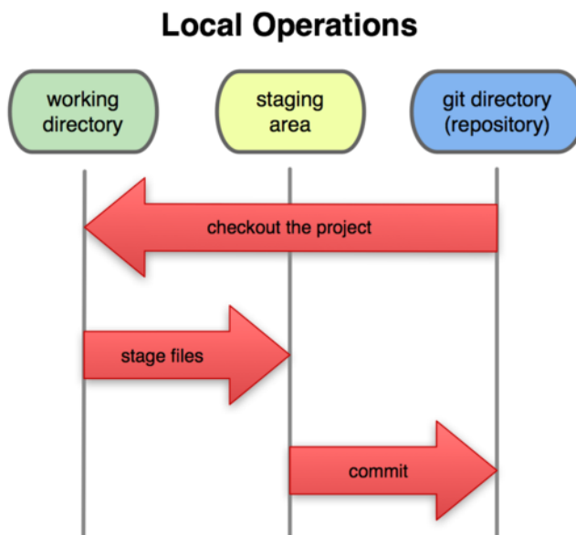
Figure 1.6: Répertoire de travail, zone d'index et répertoire Git.
