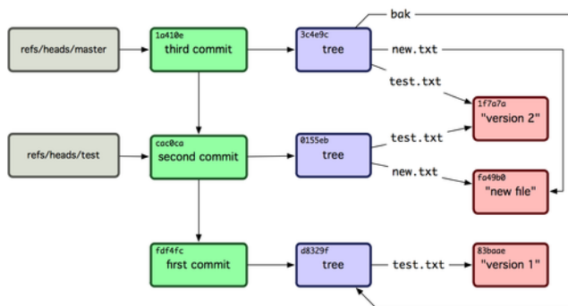
Figure 9.4: Le répertoire d'objet de Git y compris la référence au dernier état de la branche.
