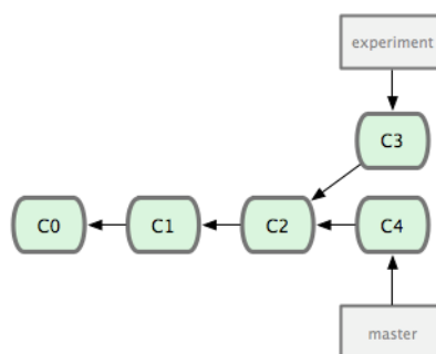
Figure 3.27: Votre historique divergent initial.
